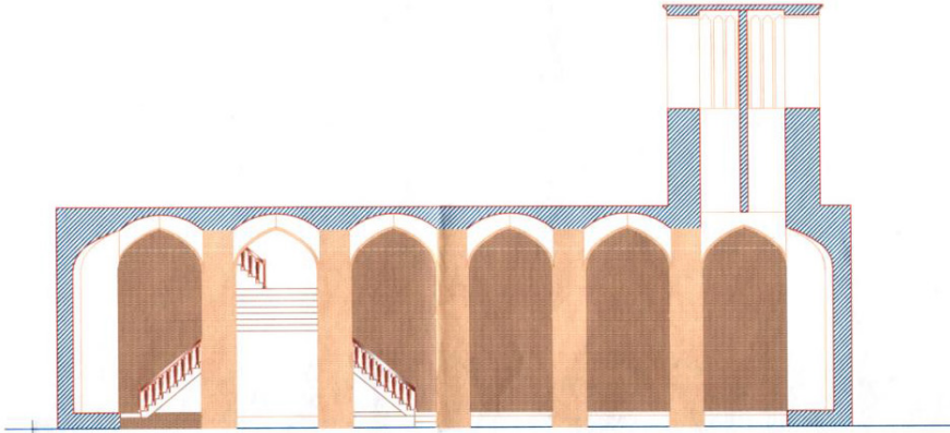
۳. برش عمودی از آب انبار سید اسماعیل (گزارش ثبتی: آب انبار سید اسماعیل، اردیبهشت ۸۵).
