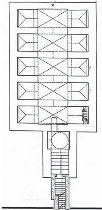
طرح شماره ۱: پلان آب انبار شیخ علیخان زنگنه اسدآباد
