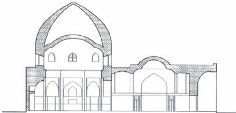
مقطع AA طرح شماره ۲: امامزاده شاهزاده حسین همدان بر گرفته از: آرشیو سازمان میراث فرهنگی استان همدان
