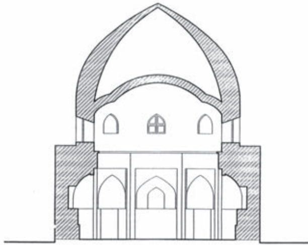
مقطع B.B طرح شماره ۳: امامزاده شاهزاده حسین همدان برگرفته از: آرشیو سازمان میراث فرهنگی استان همدان
