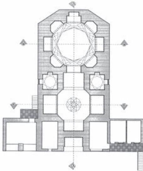
پلان شماره ۱: طبقه همکف امامزاده شاهزاده حسین همدان بر گرفته از: آرشیو سازمان میراث فرهنگی استان همدان
